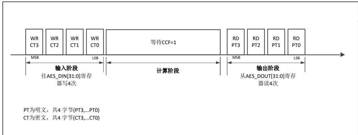
图 14-16 模式 4 示意图
