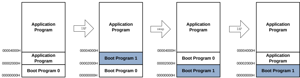
图 7-4Bootswap 示意图
