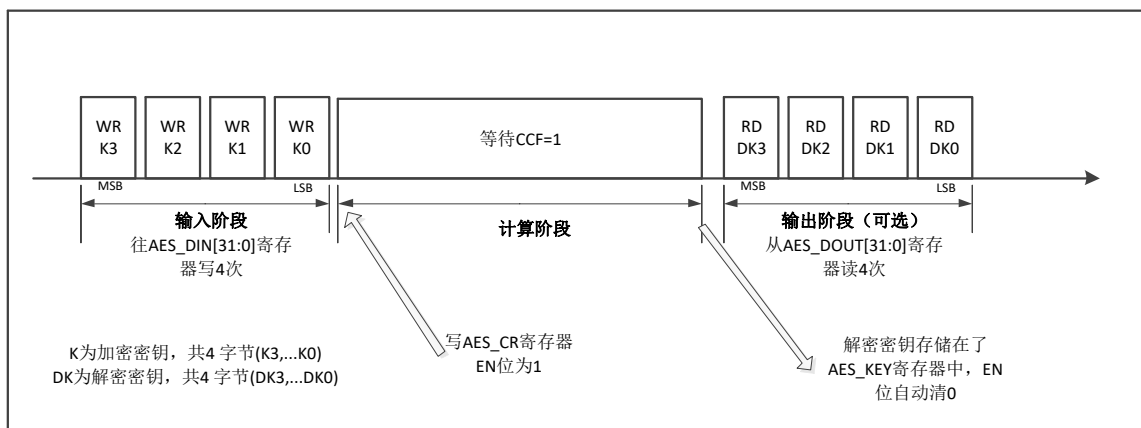
图 14-14 模式 2 示意图
