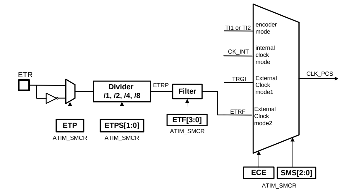
图 27-20 外部触发输入框图
