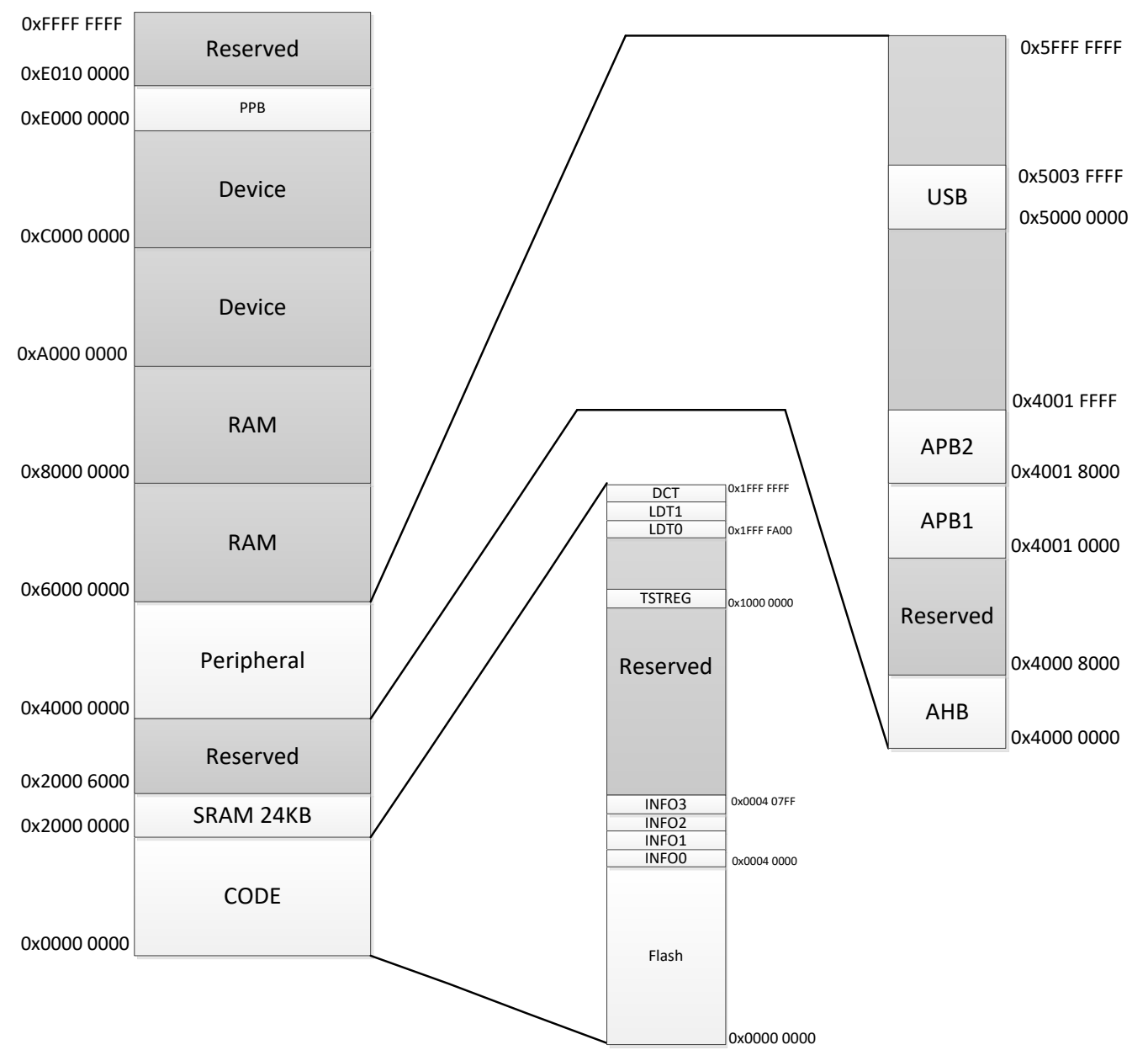
图 7-2FM33LC04x 总线地址
