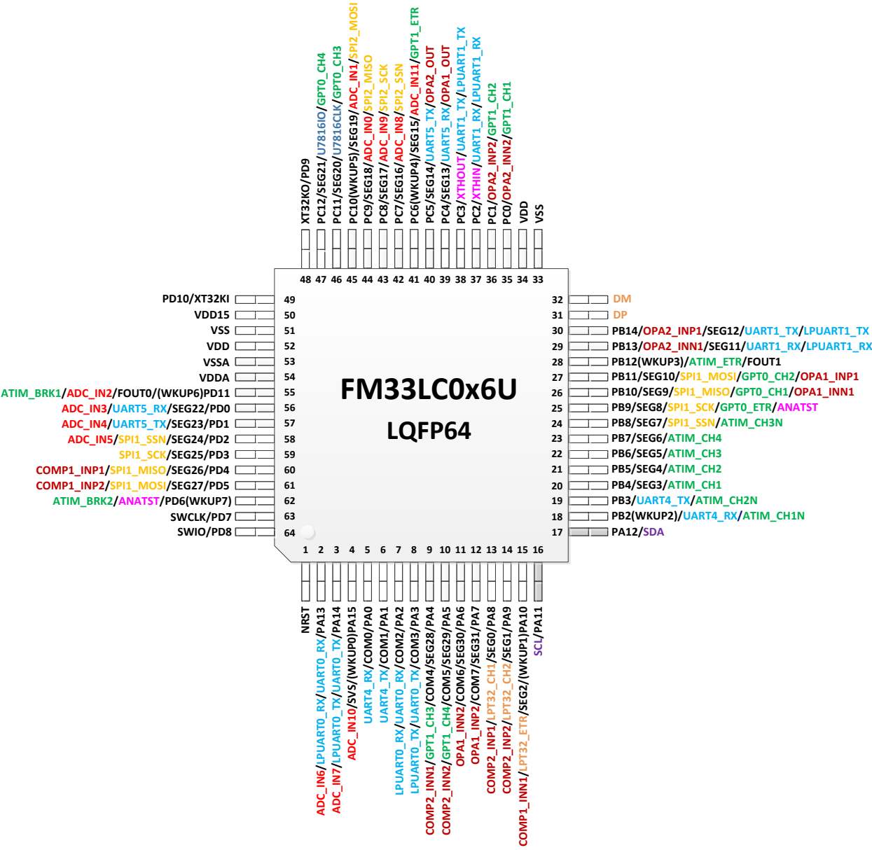
图 2-1FM33LC0x6U LQFP64 封装图
