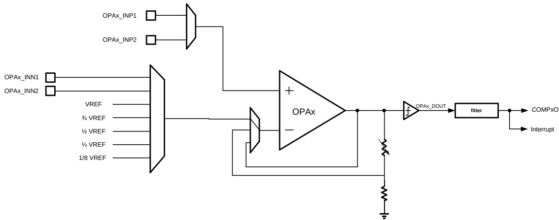
图 16-5OPA 比较器模式
