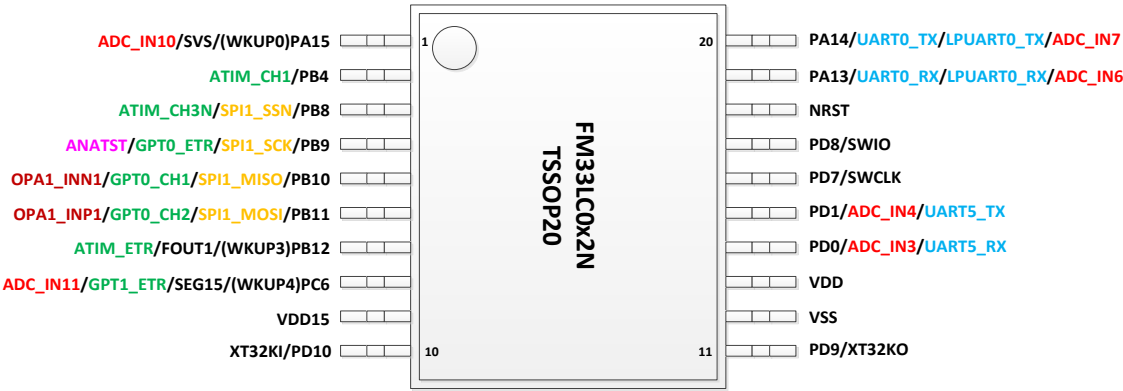
图 2-7FM33LC0x3NTSSOP20 封装图
