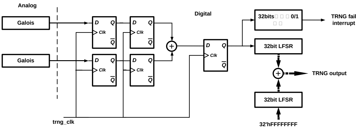
图 15-1 真随机数模块框图
