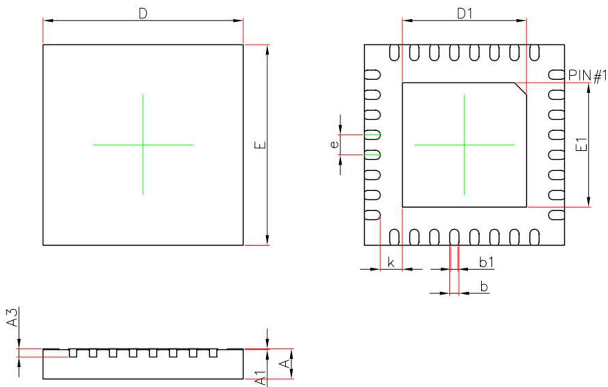
图 2-11QFN32 封装尺寸图
