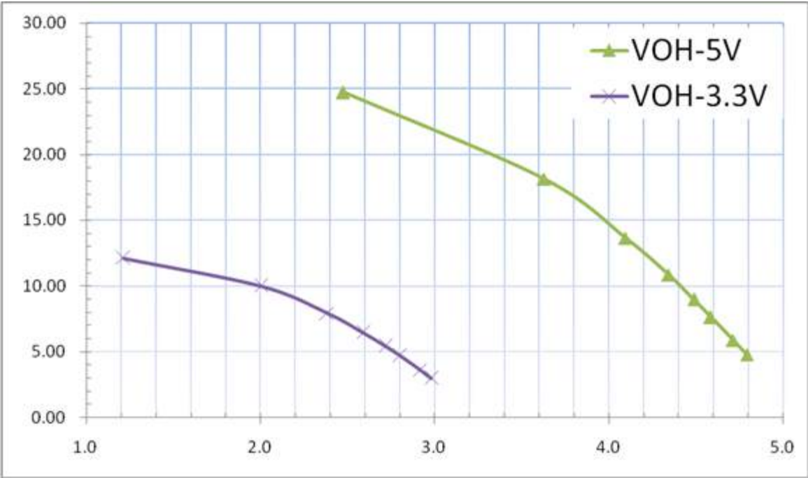
真开漏 IO（PA11、PA12）
