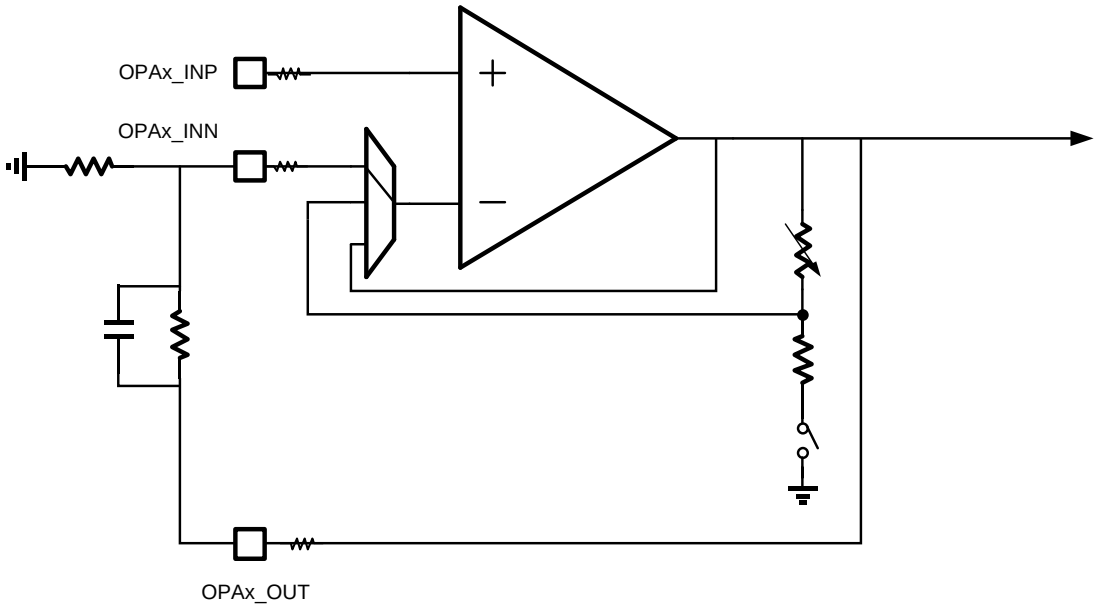
图 16-4OPA 独立模式
