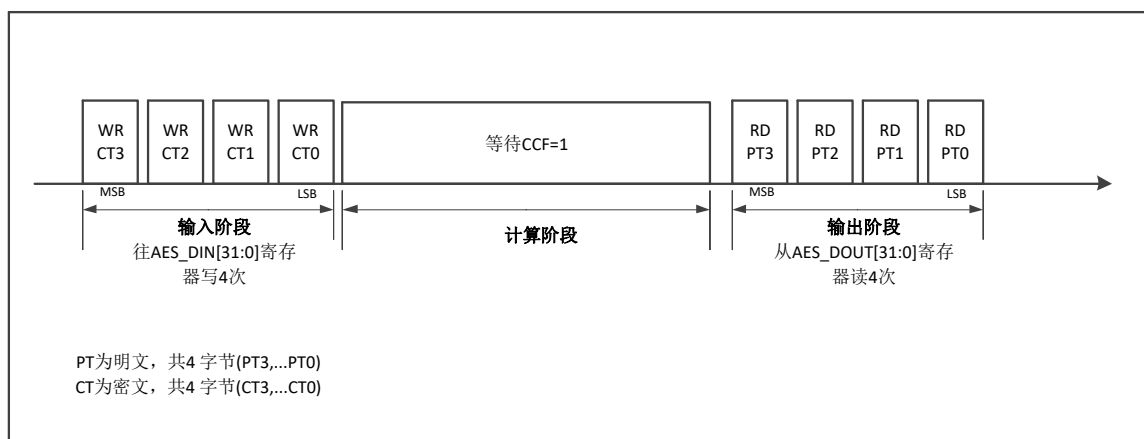
图 14-15 模式 3 示意图
