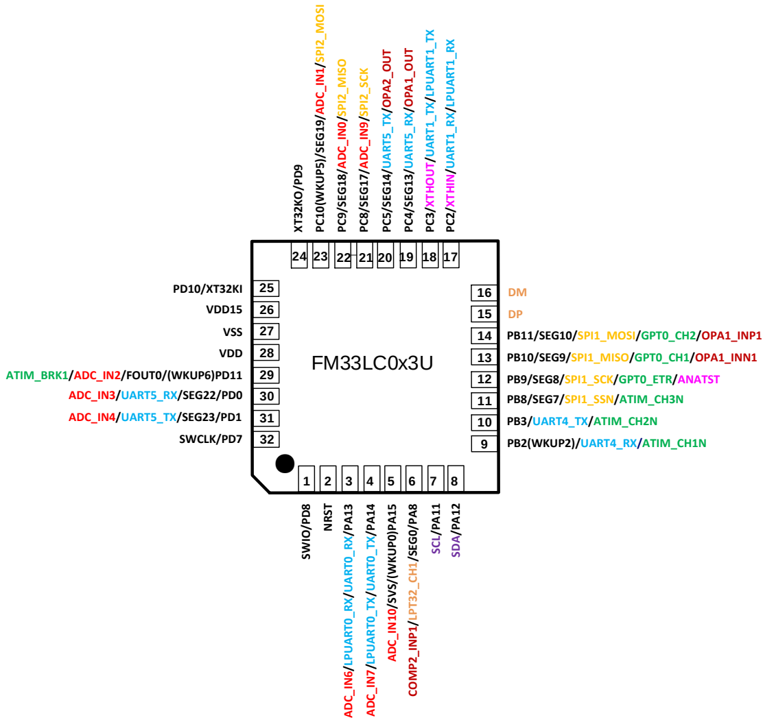
图 2-6FM33LC0x3U QFN32 封装图
