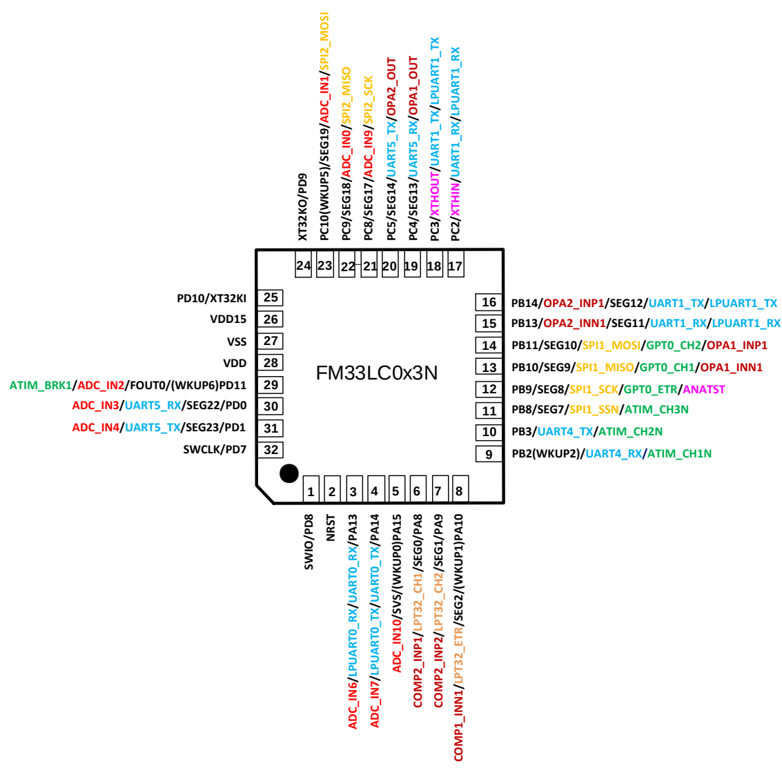
图 2-5FM33LC0x3NQFN32 封装图
